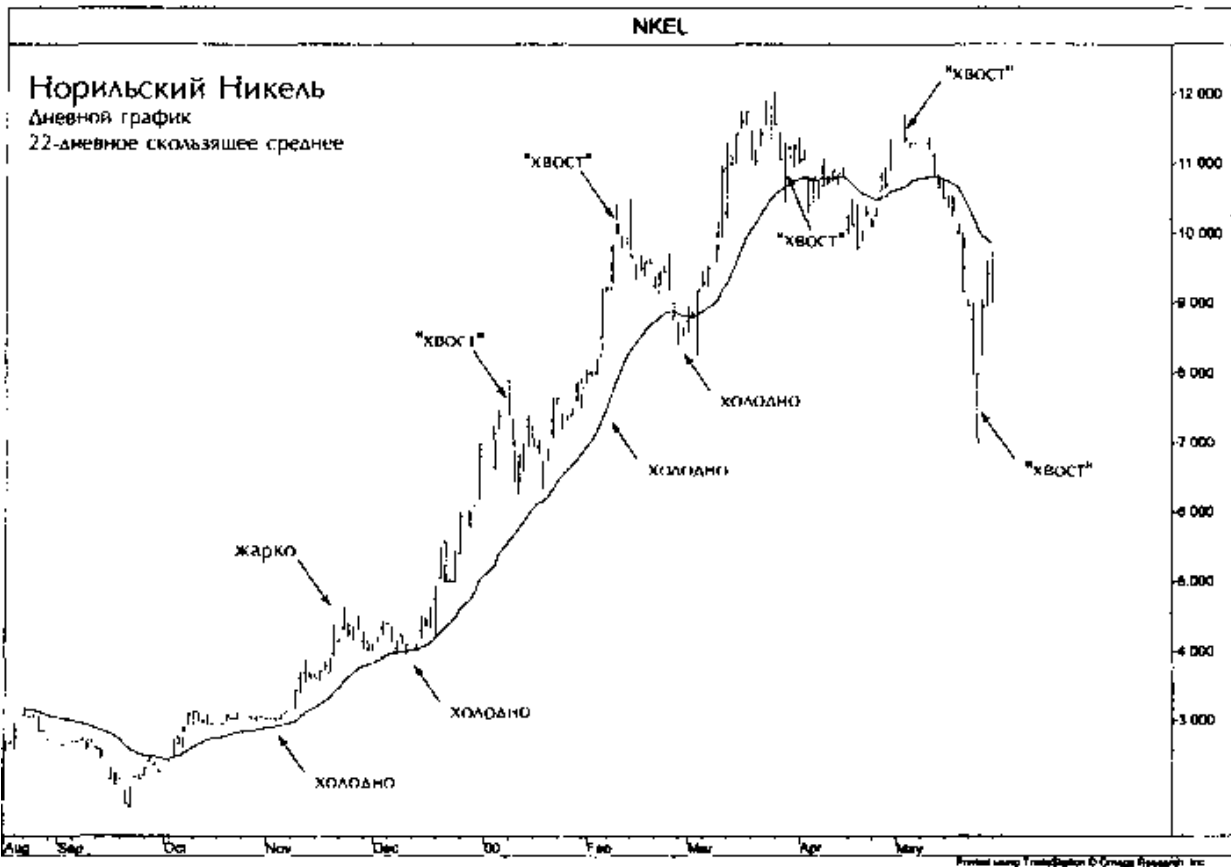
рис.1. Температура, хвосты, скользящее среднее.
